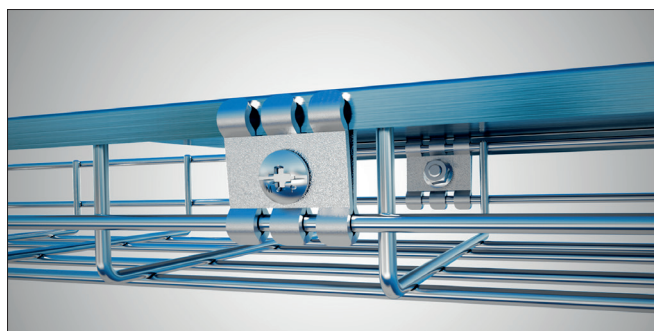
Montering av lokk med universalbrikke.
